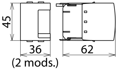
Dimension drawing DSE MOD PE 60
