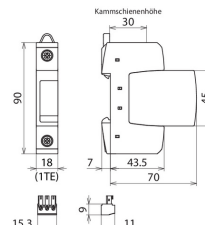
Rozměry DG S ACI 385 FM
