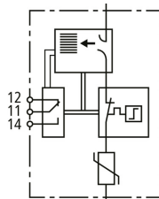
Schéma vnitřního zapojení DG S ACI 385 FM
