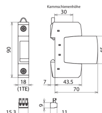
Rozměry DG S ACI 275 FM
