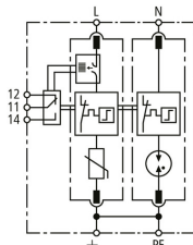
Schéma vnitřního zapojení DG M TN ACI 275 FM
