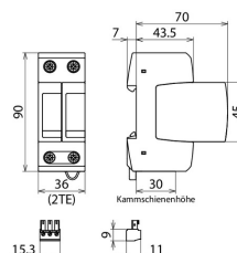
Rozměry DG M TN ACI 275 FM
