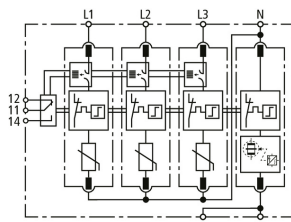
Schéma vnitřního zapojení DG M TT ACI 385 FM
