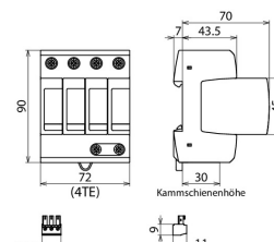
Rozměry DG M TT ACI 385 FM
