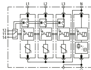
Schéma vnitřního zapojení DG M TT ACI 275 FM
