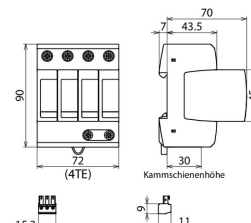
Rozměry DG M TT ACI 275 FM
