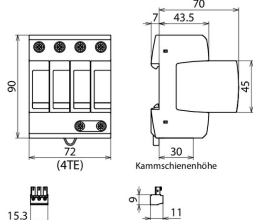
Rozměry DG M TNS ACI 275 FM
