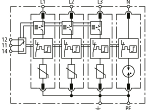
Schéma vnitřního zapojení DG M TNS ACI 275 FM
