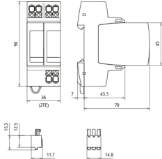
Rozměry DG MP TT 2P ACI 385 FM
