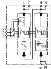
Schéma vnitřního zapojení DG MP TT 2P ACI 275 FM
