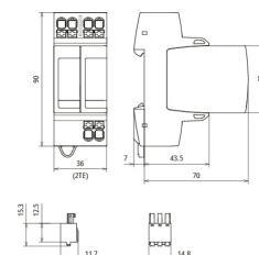
Rozměry DG MP TN ACI 275 FM
