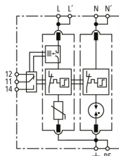
Schéma vnitřního zapojení DG MP TN ACI 275 FM
