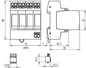
Rozměry DG MP TT ACI 385 FM
