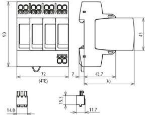
Rozměry DG MP TT ACI 275 FM
