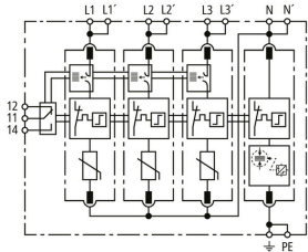
Schéma vnitřního zapojení DG MP TT ACI 275 FM
