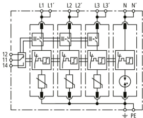
Schéma vnitřního zapojení DG MP TNS ACI 275 FM
