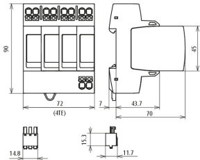
Rozměry DG MP TNS ACI 275 FM
