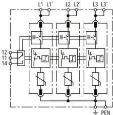
Schéma vnitřního zapojení DG MP TNC ACI 275 FM
