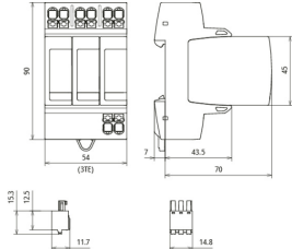
Rozměry DG MP TNC ACI 275 FM
