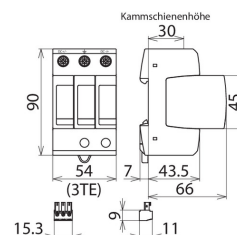
Rozměry DG M YPV SCI 1200 FM
