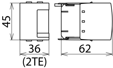
Rozměry DV MOD NPE 100
