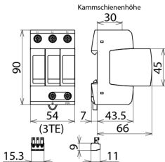
Rozměry DG M WE 600 FM
