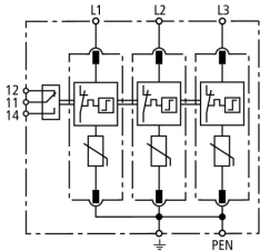
Schéma vnitřního zapojení DG M WE 600 FM
