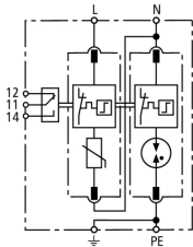
Schéma vnitřního zapojení DG M TT 2P 385 FM
