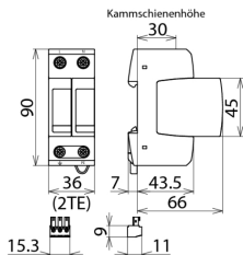
Rozměry DG M TT 2P 385 FM
