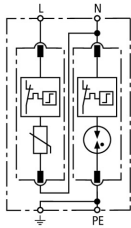
Schéma vnitřního zapojení DG M TT 2P 385
