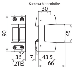
Rozměry DG M TT 2P 385
