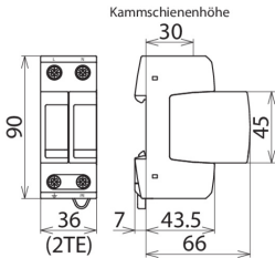
Rozměry DG M TT 2P 320
