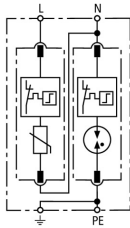
Schéma vnitřního zapojení DG M TT 2P 320
