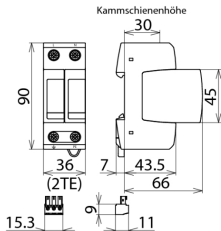
Rozměry DG M H TT 2P 275 FM
