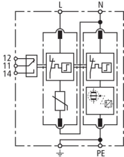
Schéma vnitřního zapojení DG M H TT 2P 275 FM
