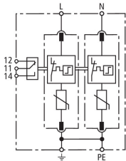
Schéma vnitřního zapojení DG M TN 150 FM
