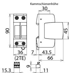
Rozměry DG M TN 150 FM
