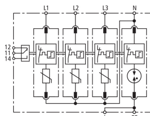
Schéma vnitřního zapojení DG M TT 385/305 FM
