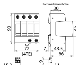
Rozměry DG M TT 385/305 FM
