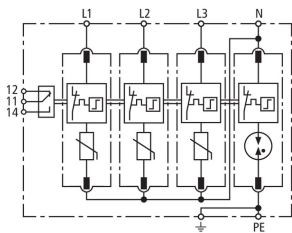
Schéma vnitřního zapojení DG M TT 385 FM
