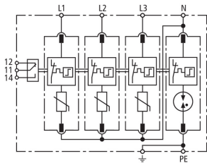
Schéma vnitřního zapojení DG M TT 320 FM
