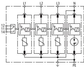
Schéma vnitřního zapojení DG M TT 150 FM
