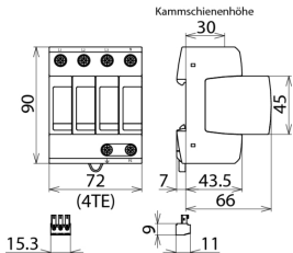
Rozměry DG M TT 150 FM
