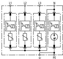
Schéma vnitřního zapojení DG M TT 385
