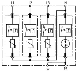
Schéma vnitřního zapojení DG M TT 320
