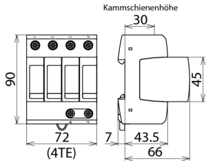
Rozměry DG M TT 320
