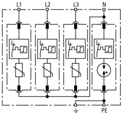
Schéma vnitřního zapojení DG M TT 275
