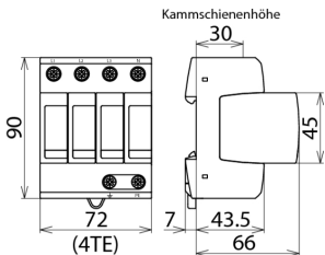
Rozměry DG M TT 275
