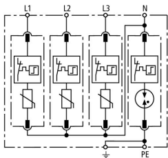
Schéma vnitřního zapojení DG M TT 150
