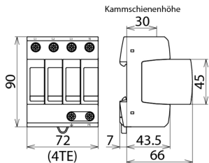
Rozměry DG M TT 150
