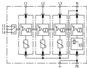
Schéma vnitřního zapojení DG M H TT 275 FM
