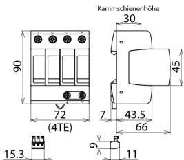
Rozměry DG M TNS 150 FM
