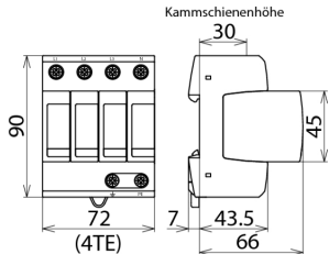
Rozměry DG M TNS 150
