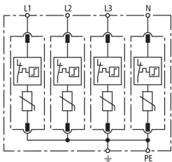
Schéma vnitřního zapojení DG M TNS 150
