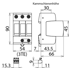
Rozměry DG M TNC 440 FM
