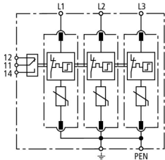
Schéma vnitřního zapojení DG M TNC 275 FM
