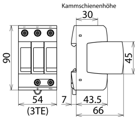
Rozměry DG M TNC 385
