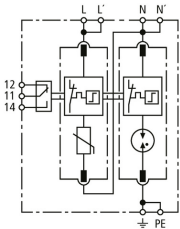
Schéma vnitřního zapojení DG MP TT 2P 320 FM
