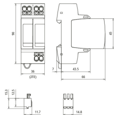
Rozměry DG MP TT 2P 320 FM
