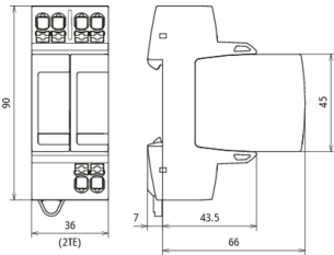
Rozměry DG MP TT 2P 275
