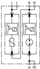
Schéma vnitřního zapojení DG MP TT 2P 275
