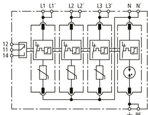
Schéma vnitřního zapojení DG MP TT 385 FM
