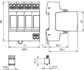
Rozměry DG MP TT 385 FM
