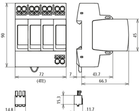
Rozměry DG MP TT 275 FM
