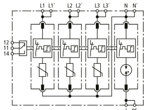
Schéma vnitřního zapojení DG MP TT 275 FM
