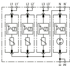
Schéma vnitřního zapojení DG MP TT 275 FM
