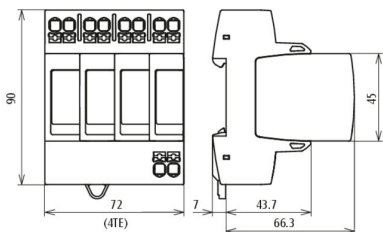
Rozměry DG MP TT 275 FM
