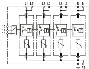
Schéma vnitřního zapojení DG MP TNS 385 FM
