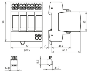
Rozměry DG MP TNS 385 FM
