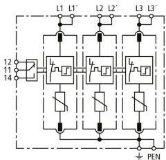
Schéma vnitřního zapojení DG MP TNC 385 FM
