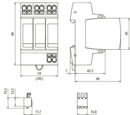
Rozměry DG MP TNC 385 FM
