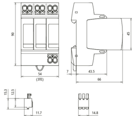
Rozměry DG MP TNC 150 FM
