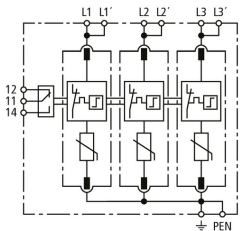
Schéma vnitřního zapojení DG MP TNC 150 FM
