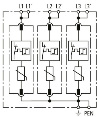
Schéma vnitřního zapojení DG MP TNC 275 FM
