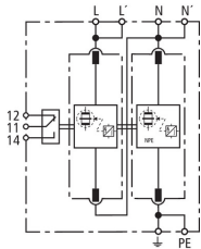
Schéma vnitřního zapojení DV M TT 2P 255 FM
