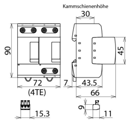
Rozměry DV M TT 2P 255 FM
