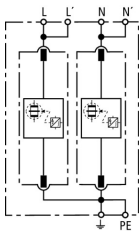
Schéma vnitřního zapojení DV M TN 255
