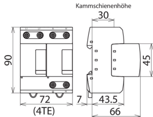
Rozměry DV M TN 255
