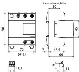
Rozměry DV M2 TNC 255 FM
