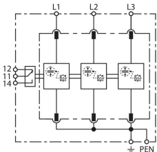
Schéma vnitřního zapojení DV M2 TNC 255 FM
