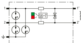
Schéma vnitřního zapojení BCO MOD ML2 EX 24
