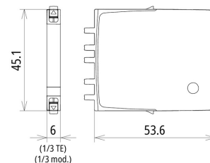
Rozměry BCO MOD ML2 BE HF 5
