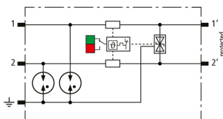
Schéma vnitřního zapojení BCO MOD ML2 BE HF 5
